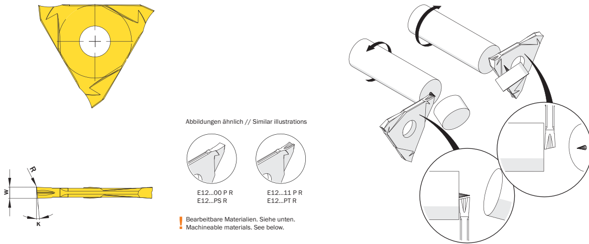
Abbildung zeigt / Drawing shows: E12.1520.11 P R
