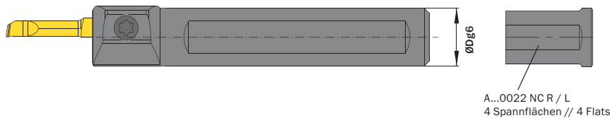
Abbildung zeigt / Drawing shows: A04.0012.NC R
