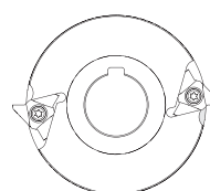
2 Plattensitze / 2 Insert seats
